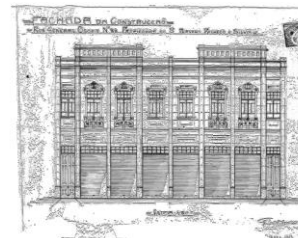
DESENHO ORIGINAL DE 1913 DA FACHADA DA CONSTRUÇÃO QUADRA 57 - Nº 383 A 490
