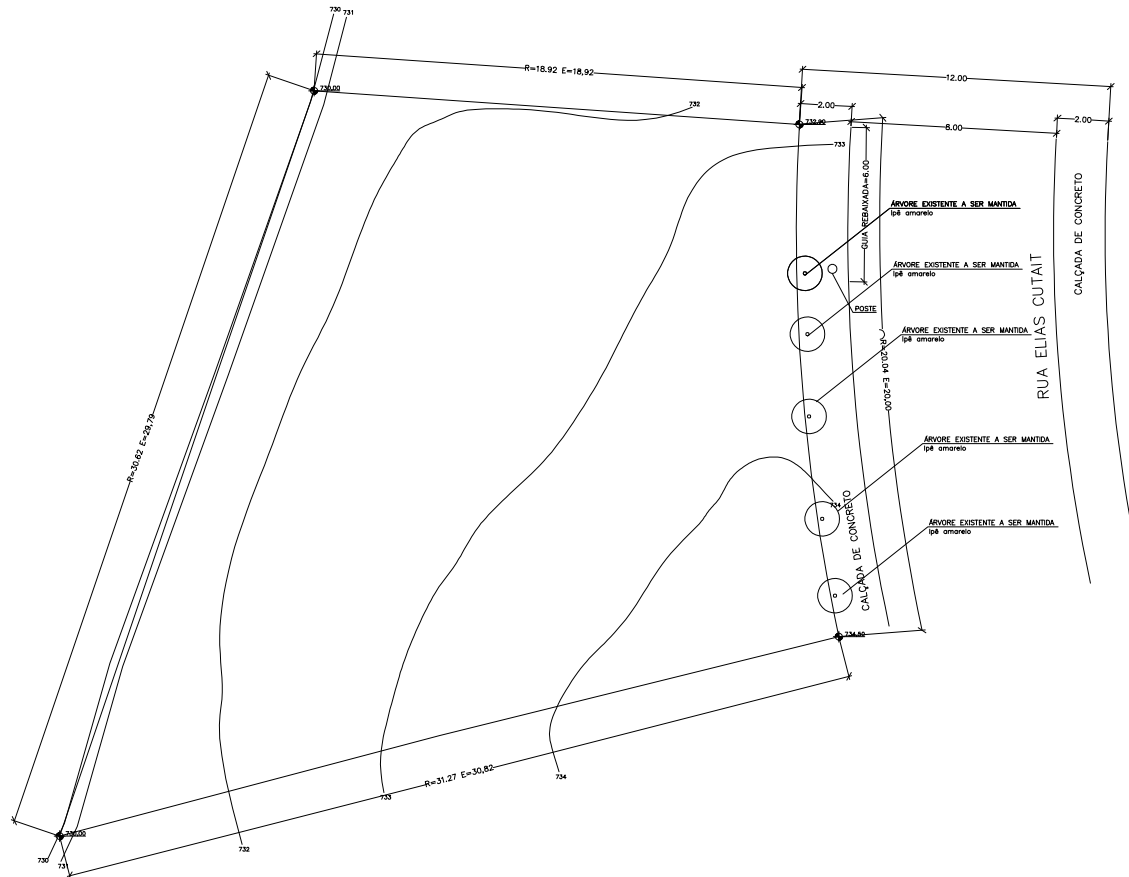
LEVANTAMENTO PLANALTIMÉTRICO ESCALA 1:100
