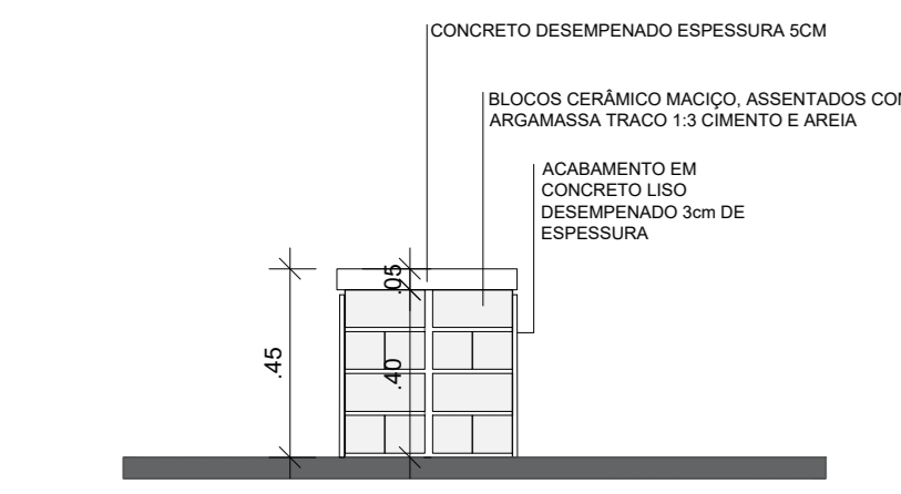
2 Detalhe tipo banco linear 1: 20
