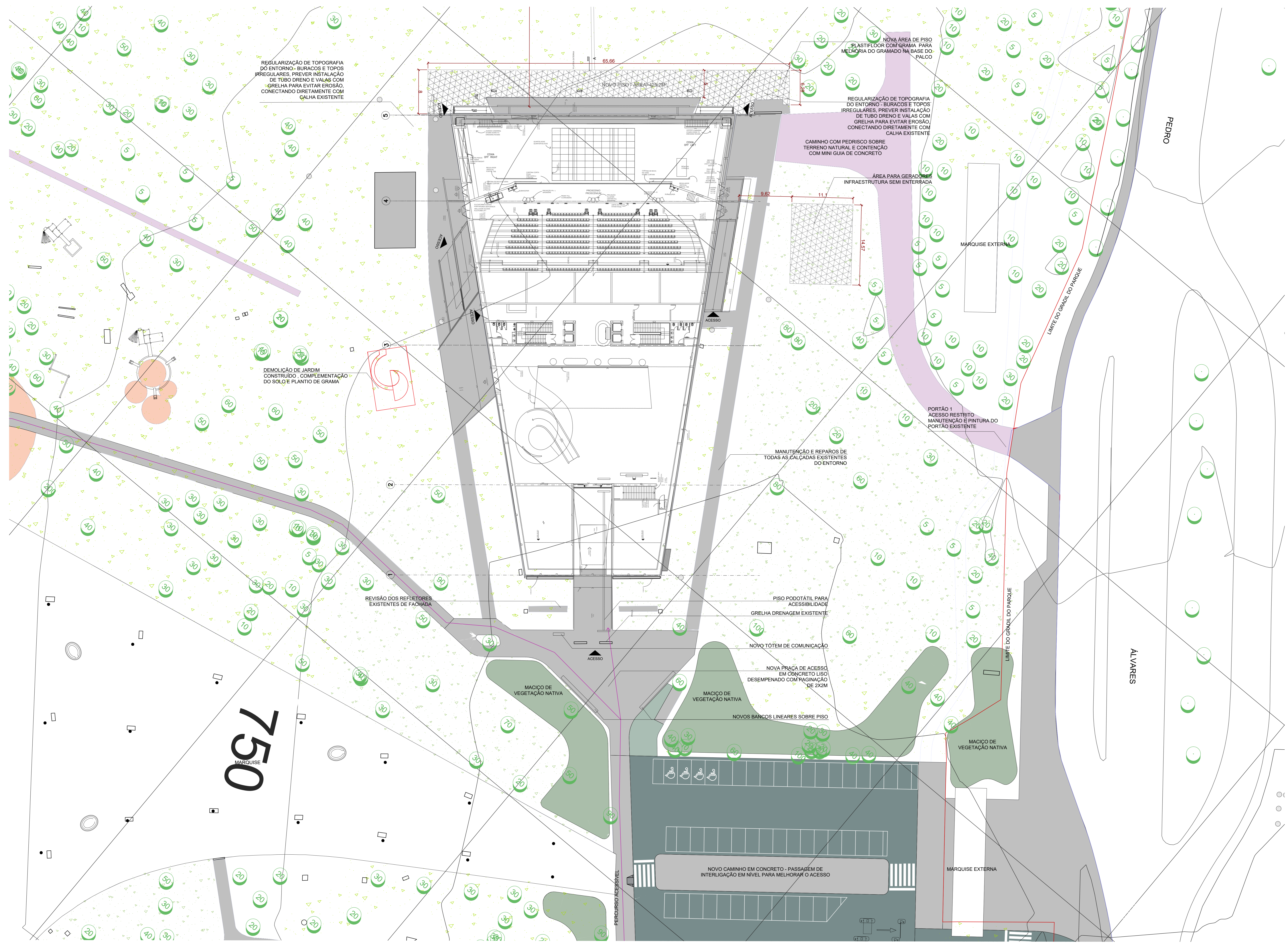
1 Implantação 1: 250
