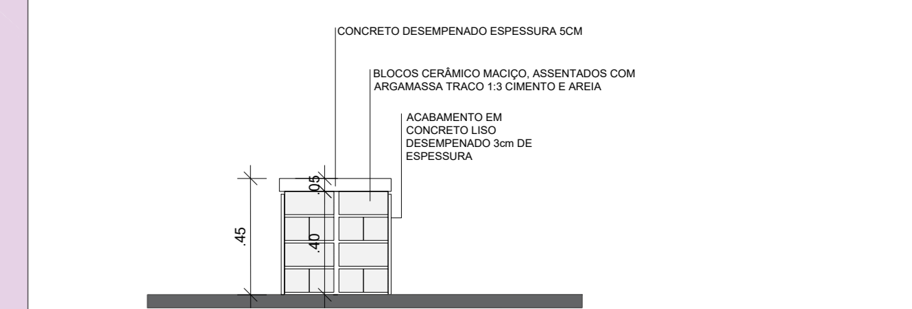
2 Banco linear 1:20
