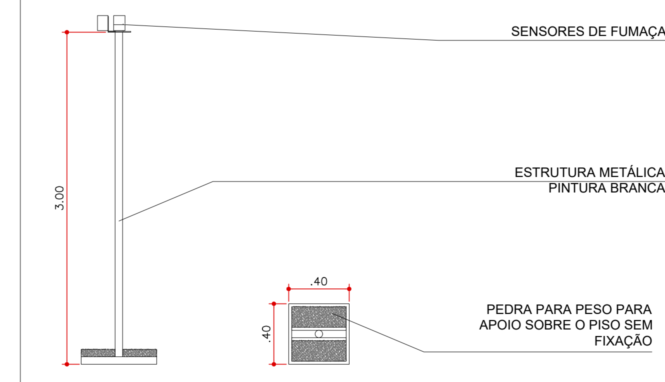
3 Postes de instalações - Corte e planta 1 : 25
