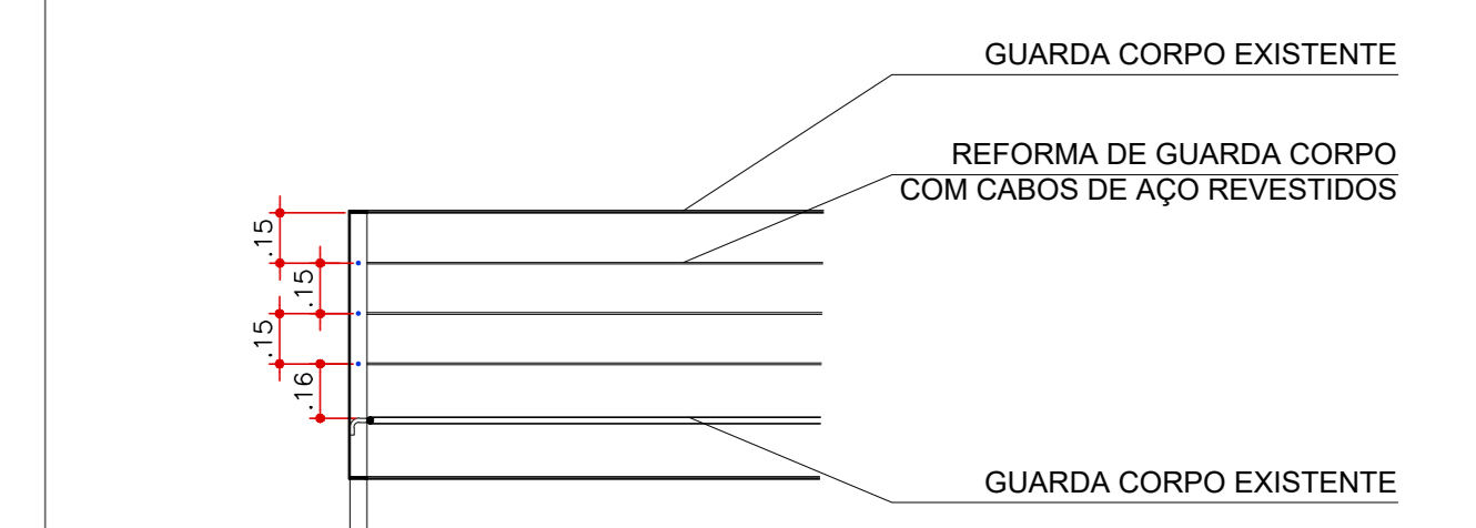
2 Corte reforma de guarda corpo 1 : 25
