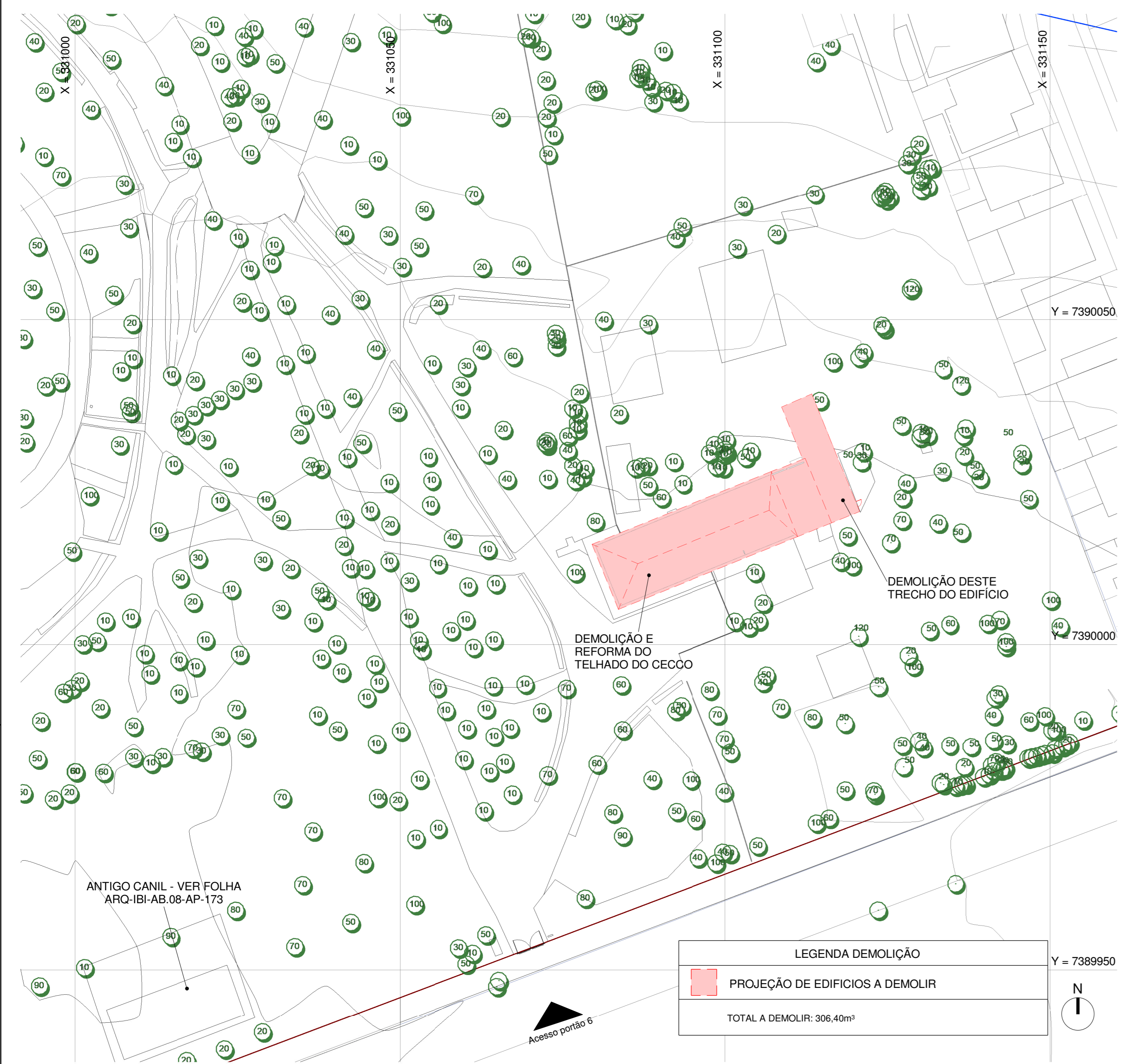
1 Planta geral de implantação e demolição 1:500
