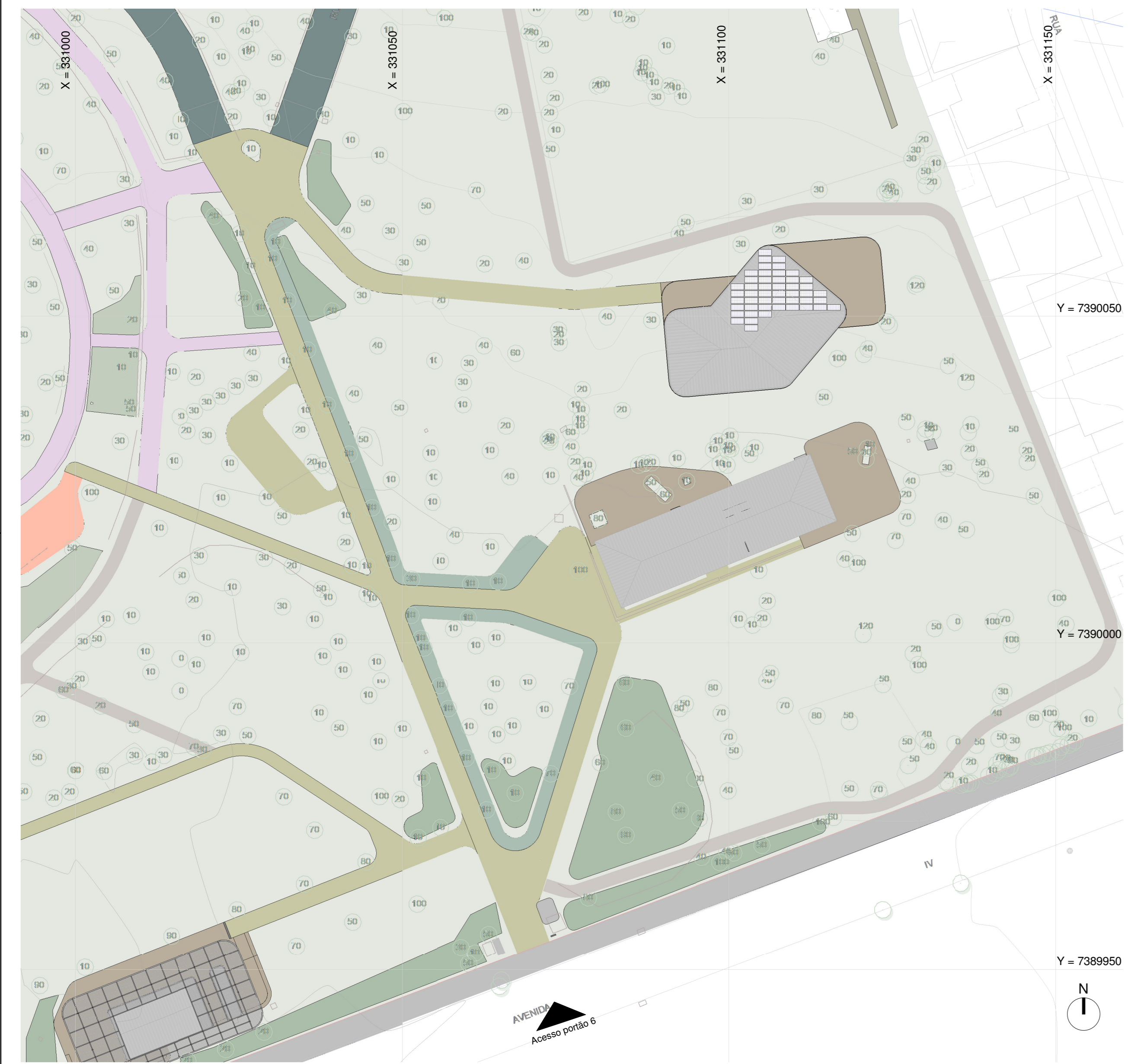
2 Implantação Geral Proposta 1:250
