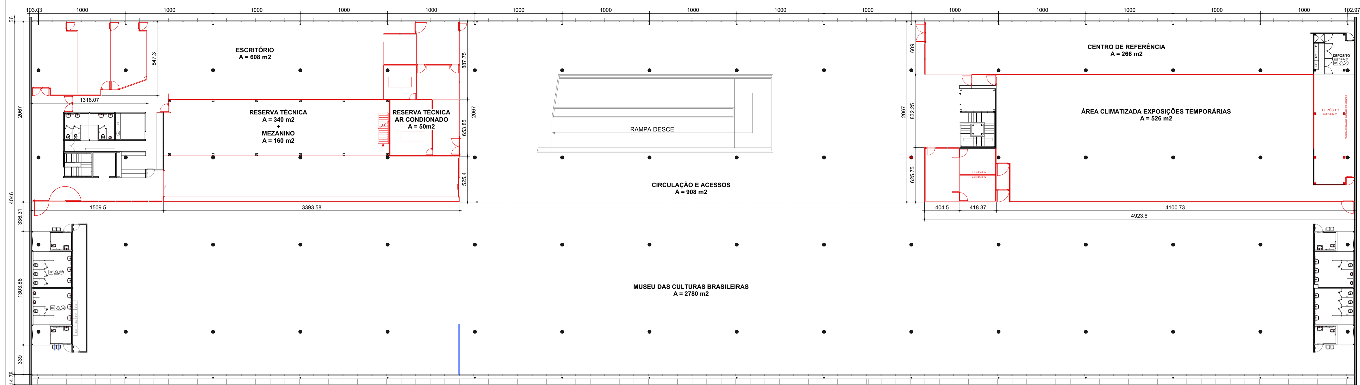
MUSEU DAS CULTURAS BRASILEIRAS | Planta - 1o pavimento | ATUAL COM INDICAÇÃO DAS REMOÇÕES esc. 1:250
