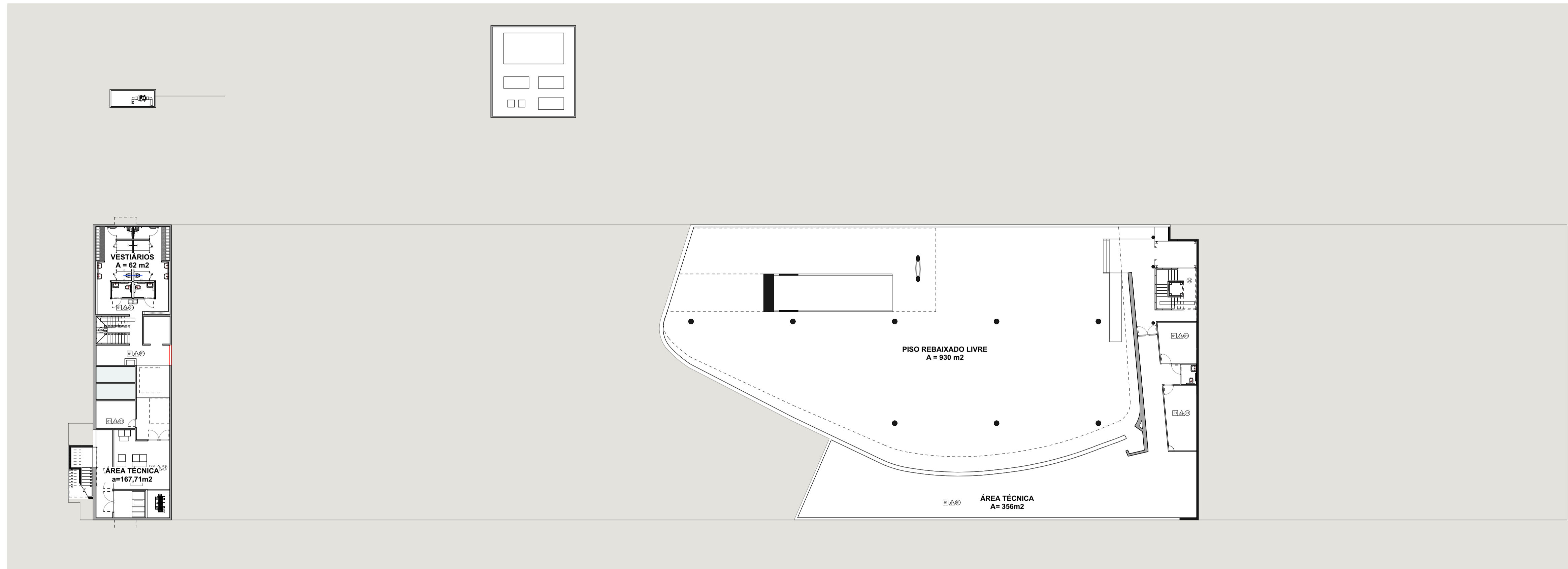
MUSEU DAS CULTURAS BRASILEIRAS | Planta - Subsolo - Existente esc. 1:250
