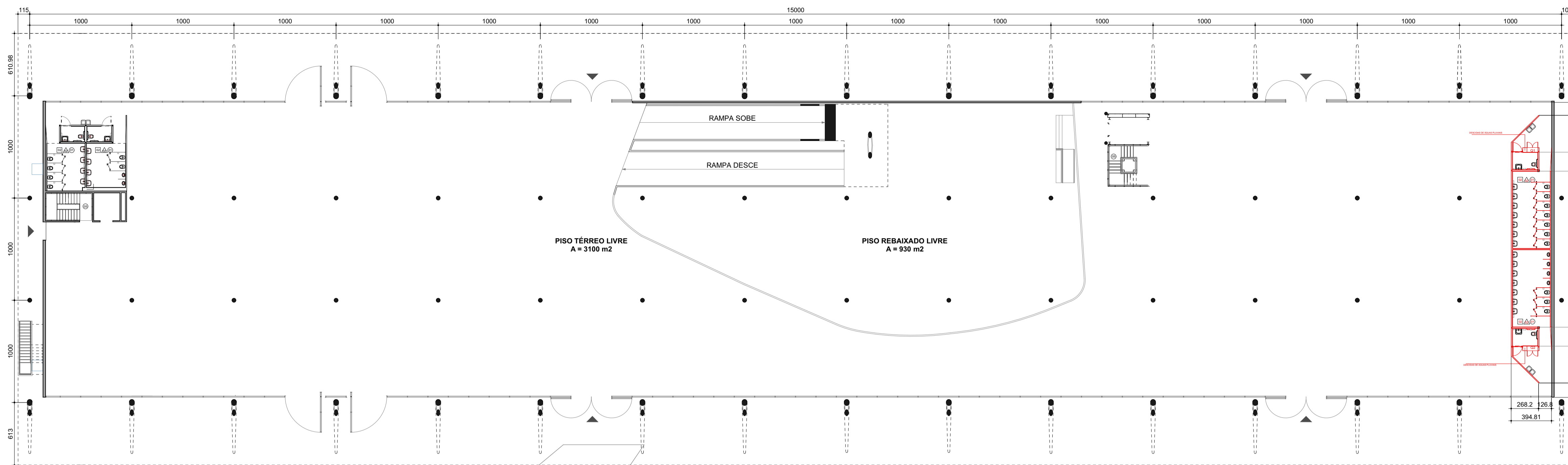
MUSEU DAS CULTURAS BRASILEIRAS | Planta - Térreo - Existente esc. 1:250
