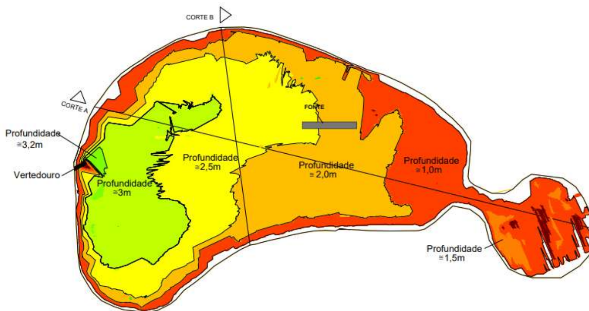
Figura 247: Batimetria do Lago das Fontes
