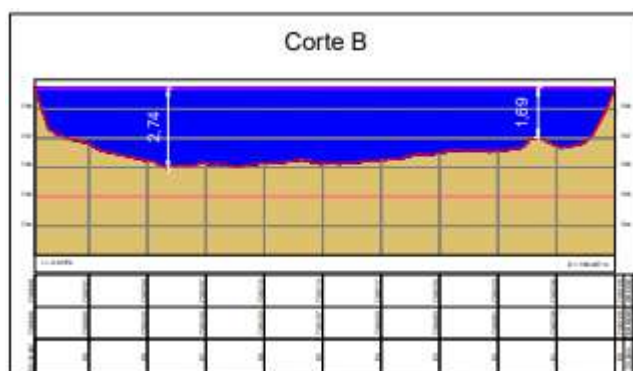
Figura 249: Batimetria do Lago das Fontes - Corte B
