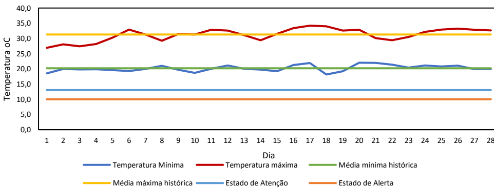
Gráfico 01. Temperaturas médias diárias mínimas e máximas, MSP, Fevereiro/2025
